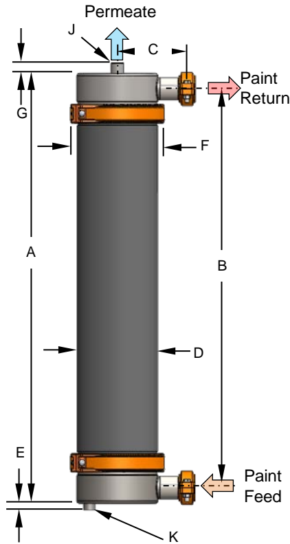
8" KPAK® PLUS Element
